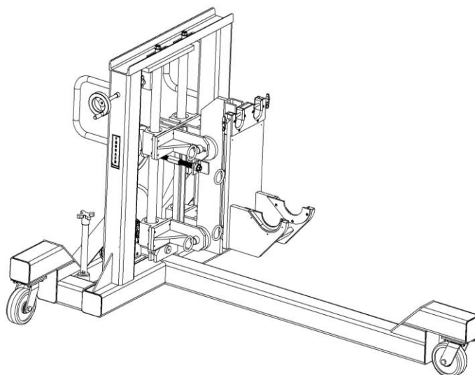
Model: 14-6930-0100 Main Landing Gear Dolly Cessna Longitude 700
